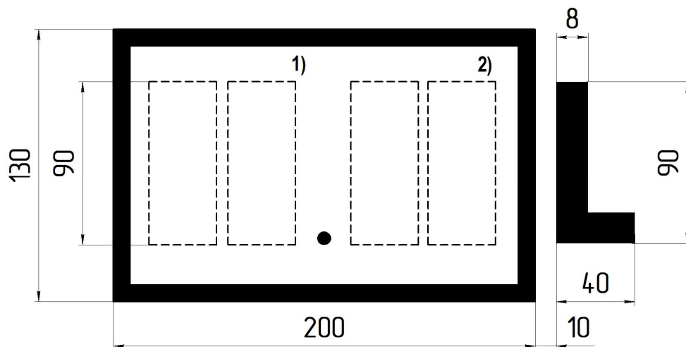
图 2：下一次定期检查罐车罐体的日期（补充 L 字符）
