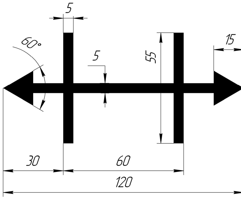
图 3：1520mm 轨距铁路附属车辆转向架的标志
