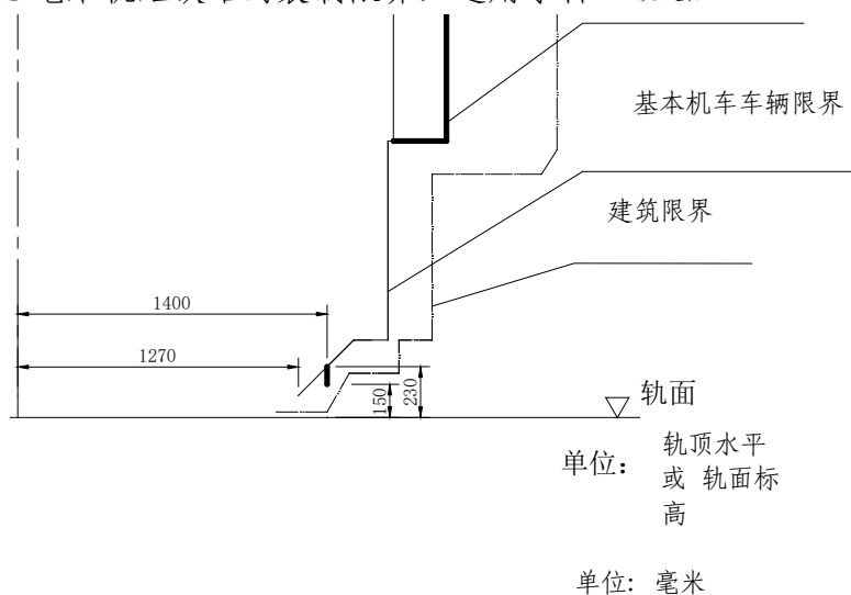
图 5b 1435 毫米轨距铁路的装载限界: 适用于科索沃铁路 (下部二级超限)
