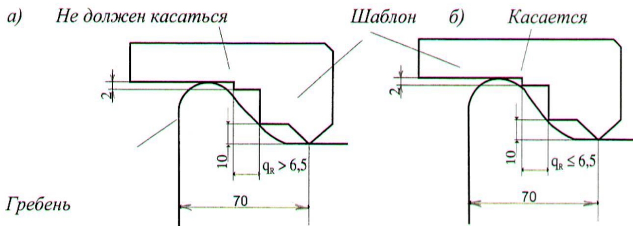
图 3：容许的轮缘 а) 和不容许的轮缘 б)
