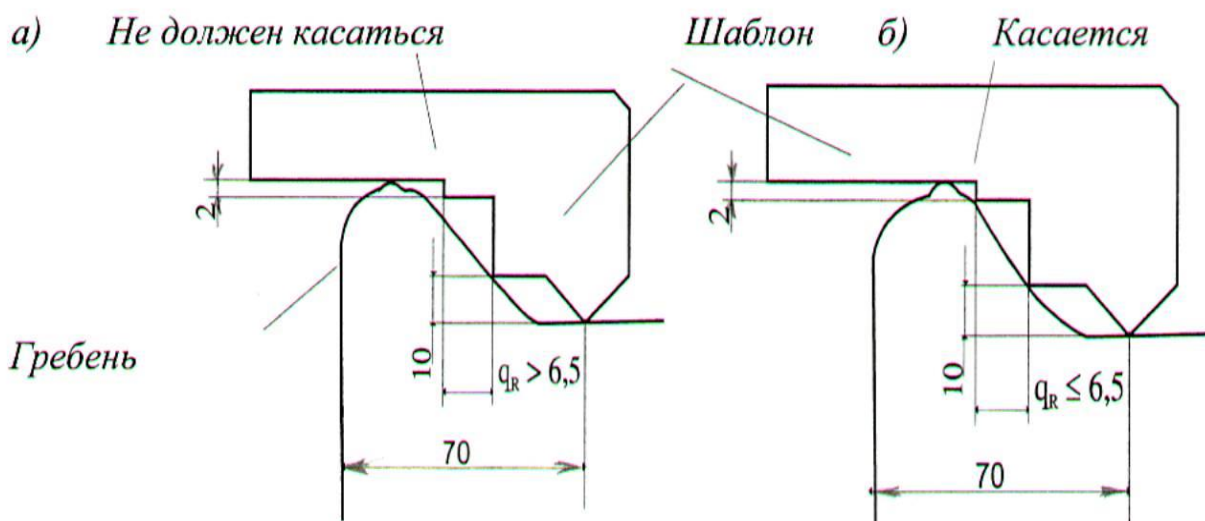
图 4：容许的轮缘 а) 和不容许的轮缘 б)
